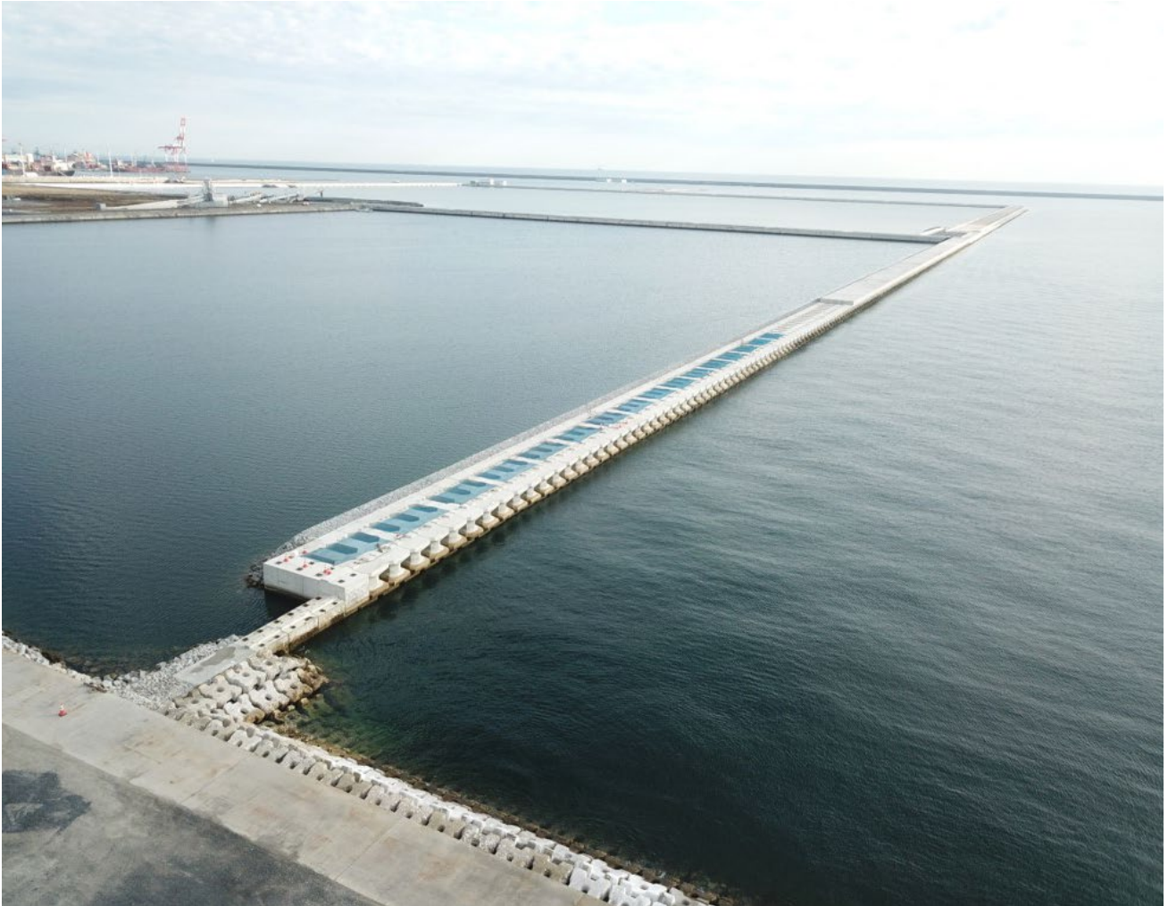
捨石法面均し管理システム活用
