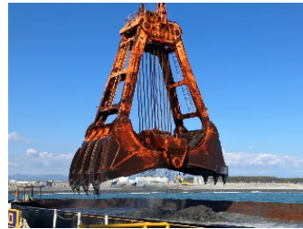
【浚渫作業③ 土砂運搬船へ土砂積込完了】
